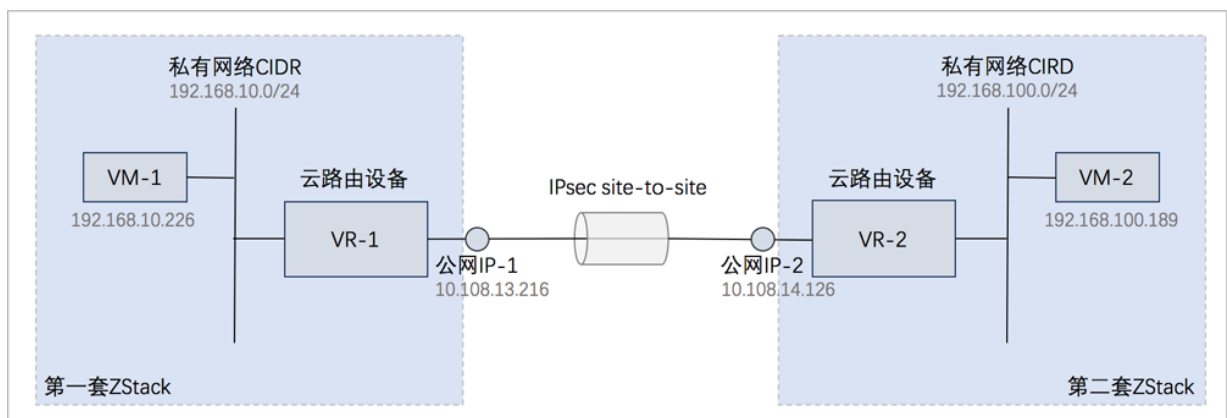
图 118: IPsec隧道网络架构图
