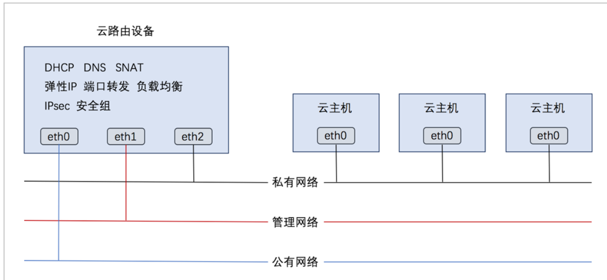
图 2: 部署方式-2
